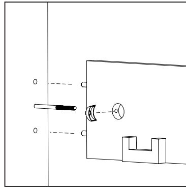
Vínculos largueros con respaldar.
